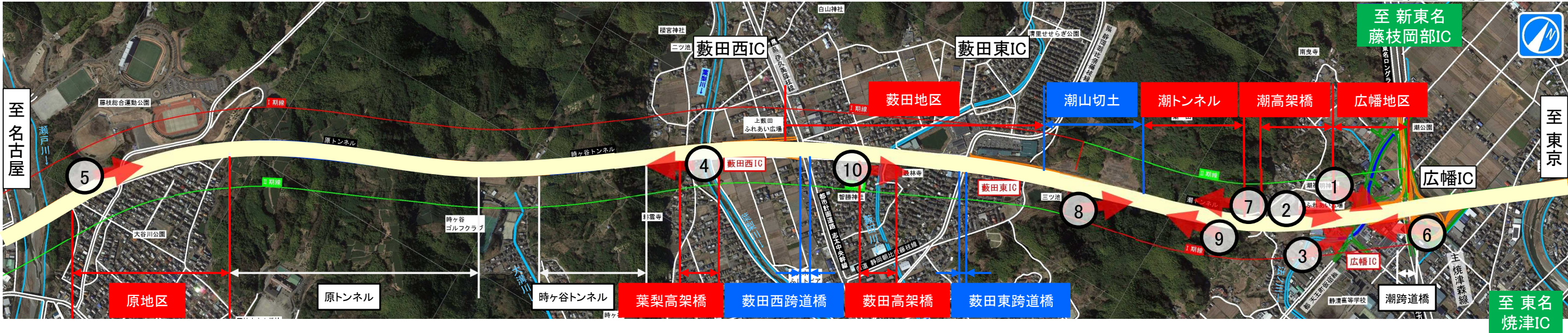
①広幡地区(本線北側) 舗装工 施工中 排水構造物工 施工完了 擁壁工 施工完了 遮音壁工 施工中
