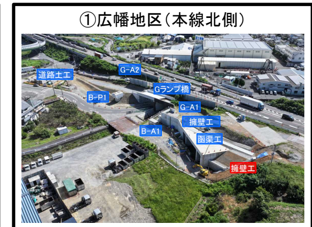
①広幡地区 (本線北側) 橋梁上部工 (Gランプ橋) 施工完了 擁壁工 施工中 遮音壁工 施工中
