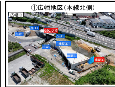
①広幡地区 (本線北側) 橋梁上部工 (Gランプ橋) 施工中 擁壁工 施工中
