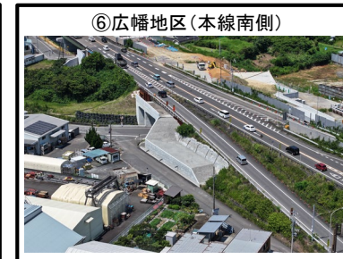
⑥広幡地区 (本線南側) 擁壁工 施工完了
