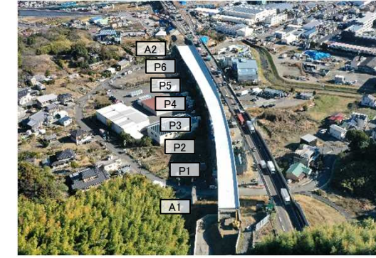
A1橋台～A2橋台 上部工 施工完了
