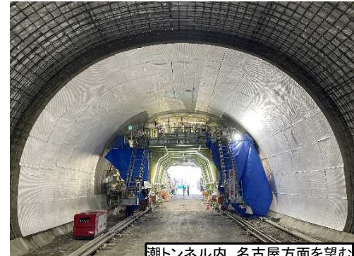
⑨潮トンネル工事（西坑口）
