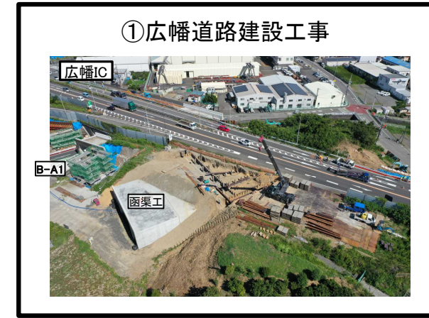
①広幡道路建設工事 天王町仮宿線 函渠工 施工中
