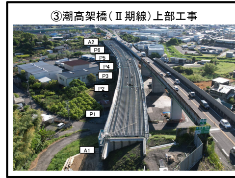
A1橋台～A2橋台 床版打設 施工中
