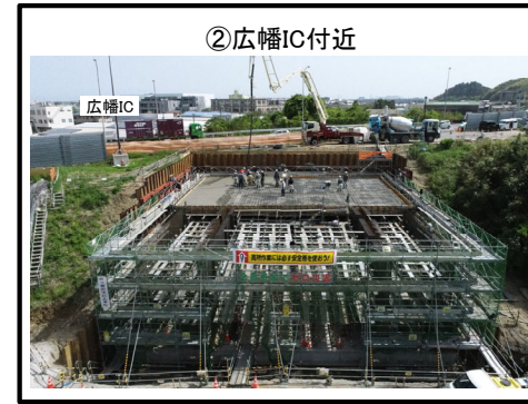
天王町仮宿線 函渠工 施工中
