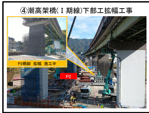
P2橋脚 下部工拡幅 施工中
