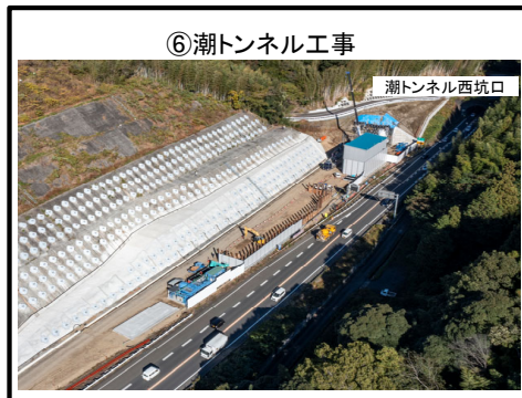
トンネル工 施工準備中
