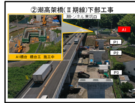
A1橋台 橋台工 施工中
