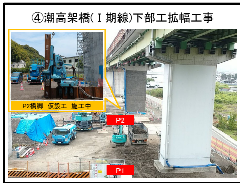
P1橋脚 P2橋脚 下部工拡幅 施工中
