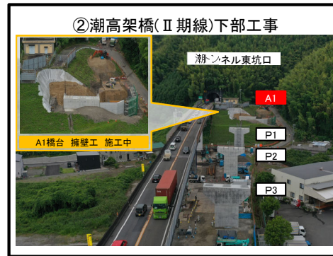
A1橋台 擁壁工 施工中
