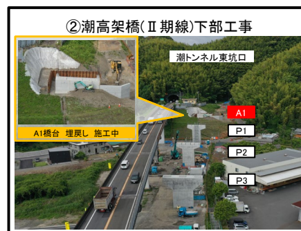
A1橋台 埋戻し 施工中
