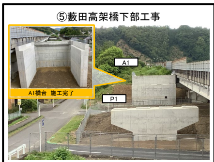
A1橋台 施工完了
