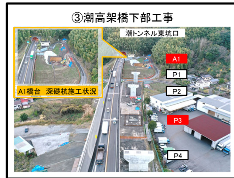
A1橋台 深礎杭工施工中
