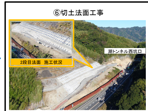
法面工 2段目施工中
