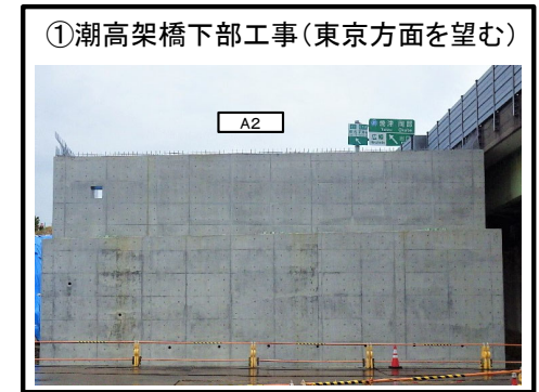
A2橋台の施工完了
