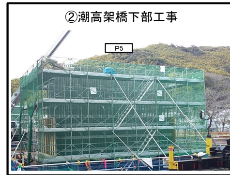
P5橋脚の柱部型枠組立中
