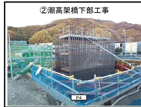
P4橋脚の柱部鉄筋組立中
