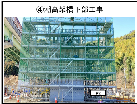
P2橋脚の柱部鉄筋組立中
