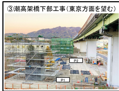
P1橋脚・P2橋脚の施工状況
