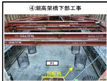
P1橋脚の杭頭処理完了
