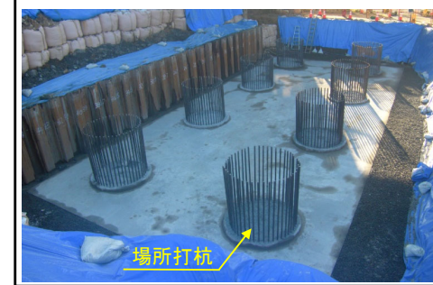
A2橋台の場所打杭施工状況(杭頭処理)
