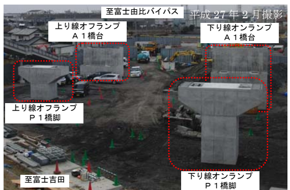
ランプ橋下部工 施工状況
