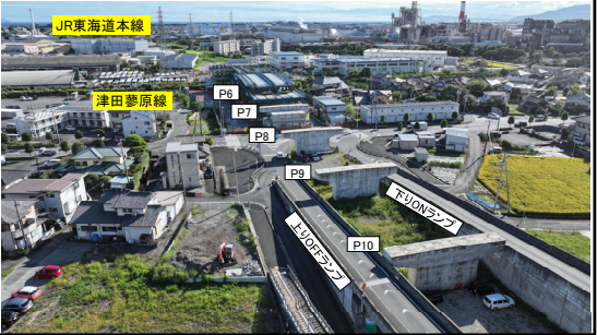
P11橋脚より南側を望む
