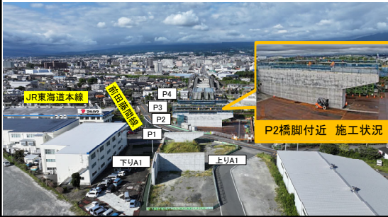
A1橋台から北側を望む
