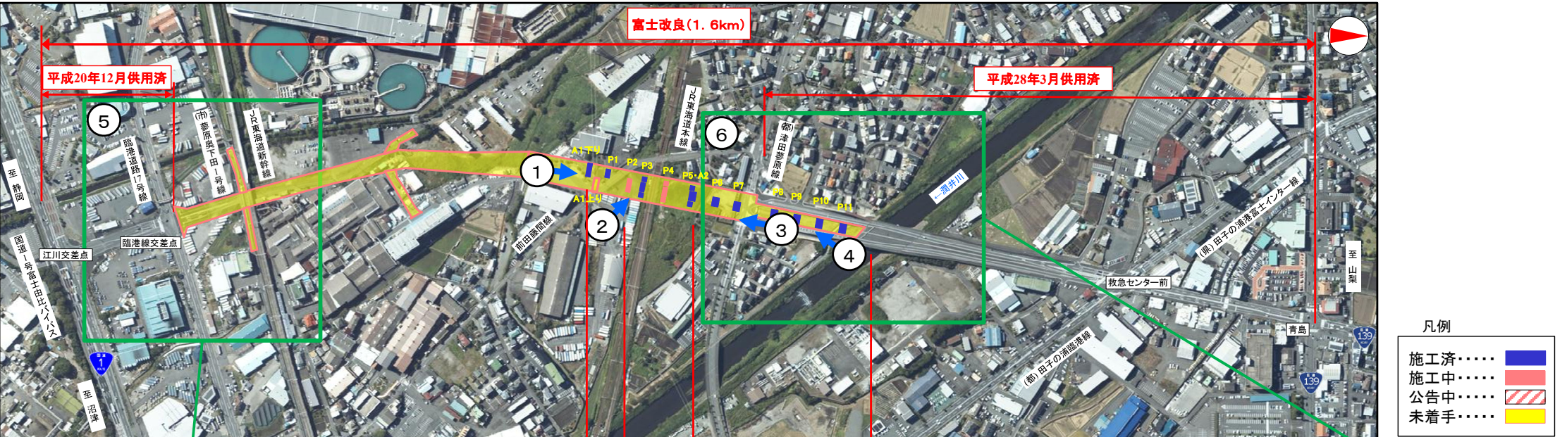
①前田地区 (No.33付近) A1橋脚 下り背面L型擁壁 施工完了
