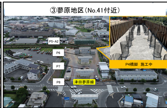
③蓼原地区 (No.41付近) P4橋脚 基礎工 施工中
