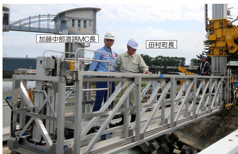
橋梁点検車にて、古川橋の近接目視点検を実施
