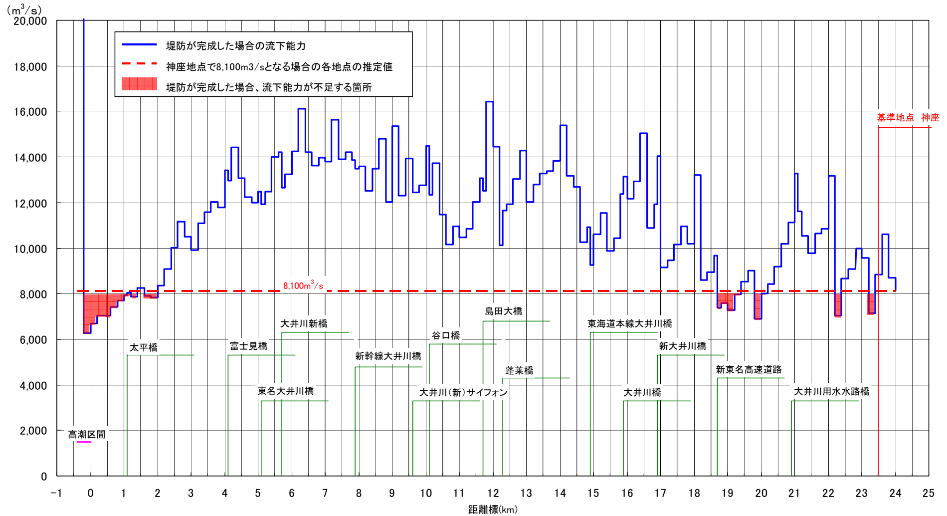
図-1.2.1 堤防が完成した場合の流下能力
