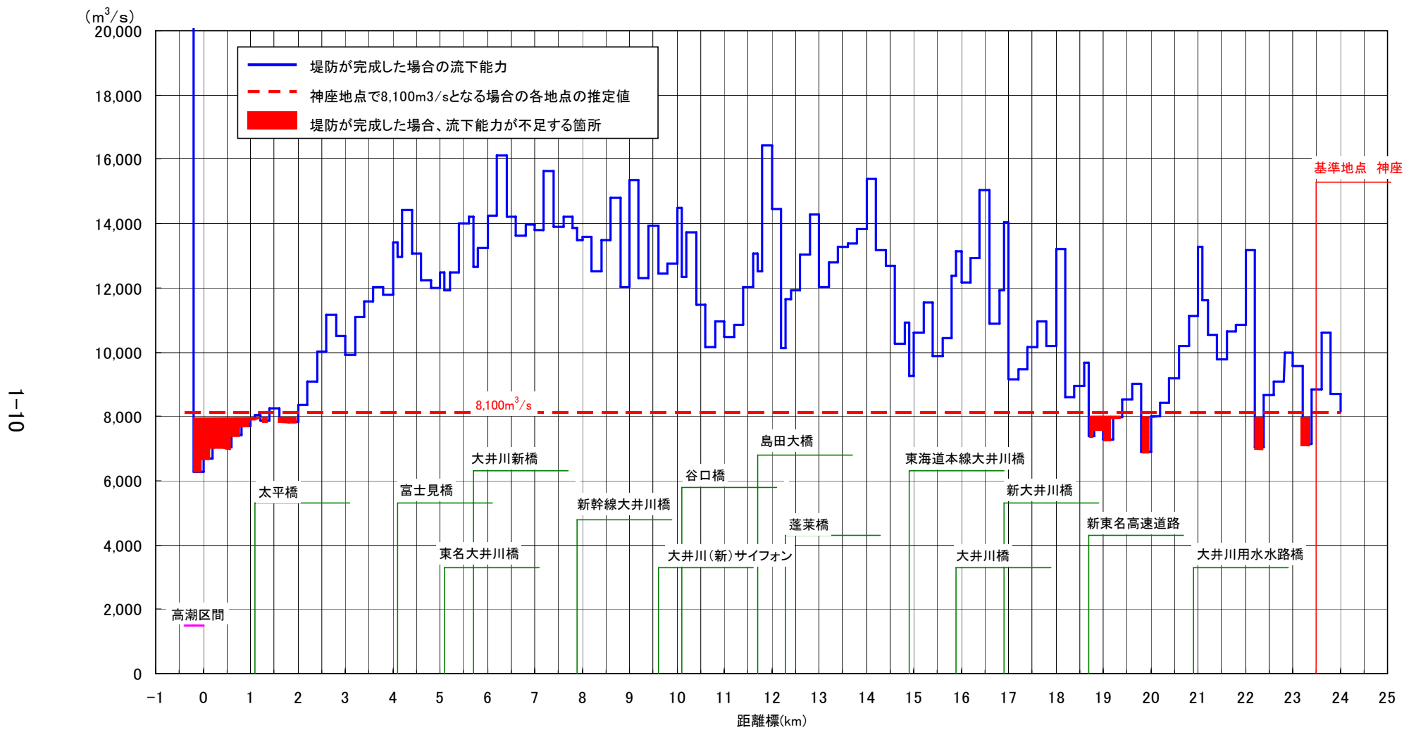
図-1.2.1 堤防が完成した場合の流下能力
