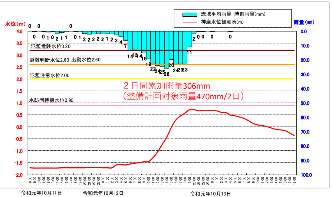
令和元年10月11日～10月13日 台風第19号による出水時の神座水位観測所の水位
