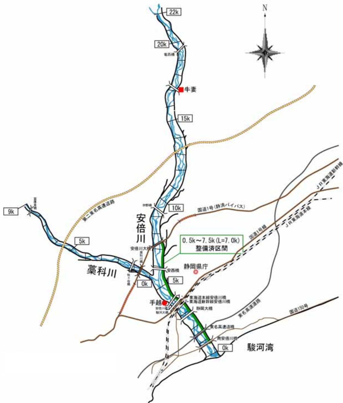
図-2.1.6 緊急用河川敷道路整備状況図
