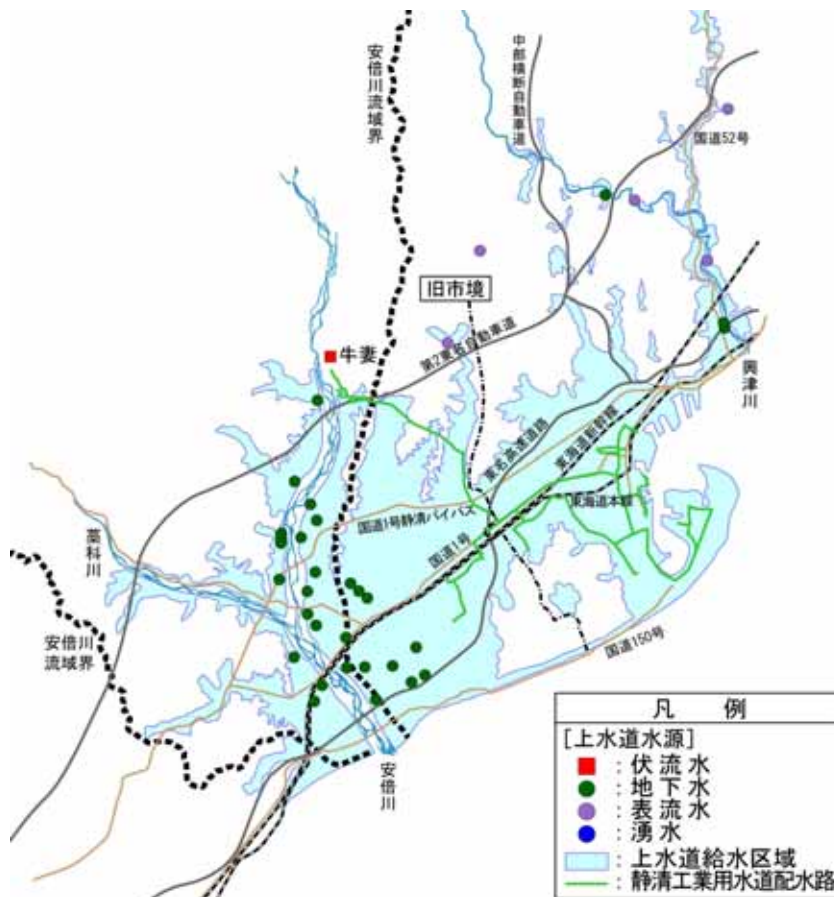
图-1.1.23 水源位置图
