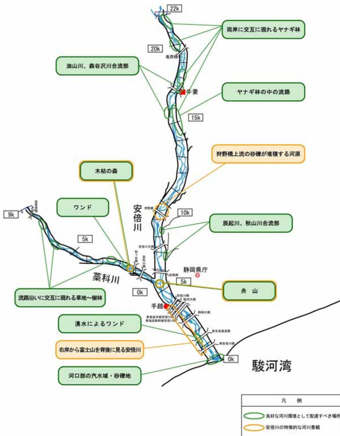
図-2.1.27 良好な河川環境として配慮すべき場所及び特徴的な河川景観の位置図
