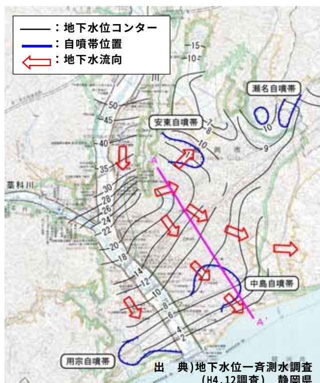
図-2.1.16 静岡平野の地下水位コンター・自噴帯位置図
