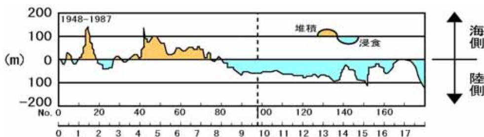
図-2.1.12 昭和 23 年（1948 年）～昭和 62 年（1987 年）の汀線変化
