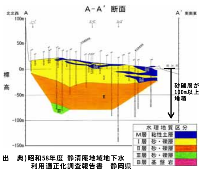
図-2.1.17 静岡平野の地質断面図
