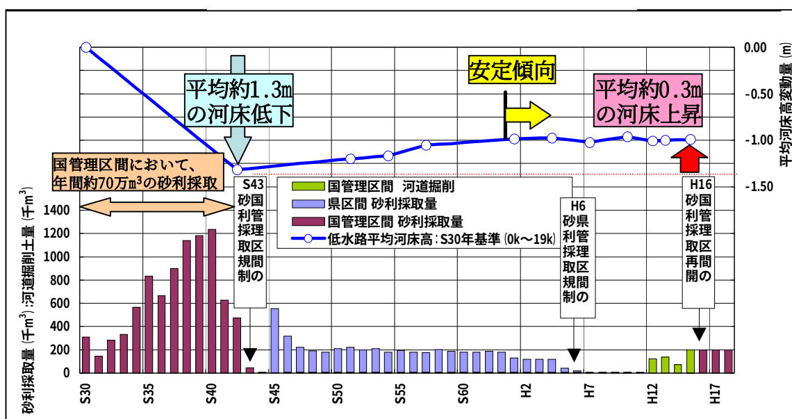
図-2.1.11 砂利採取と河床高の経年変化
