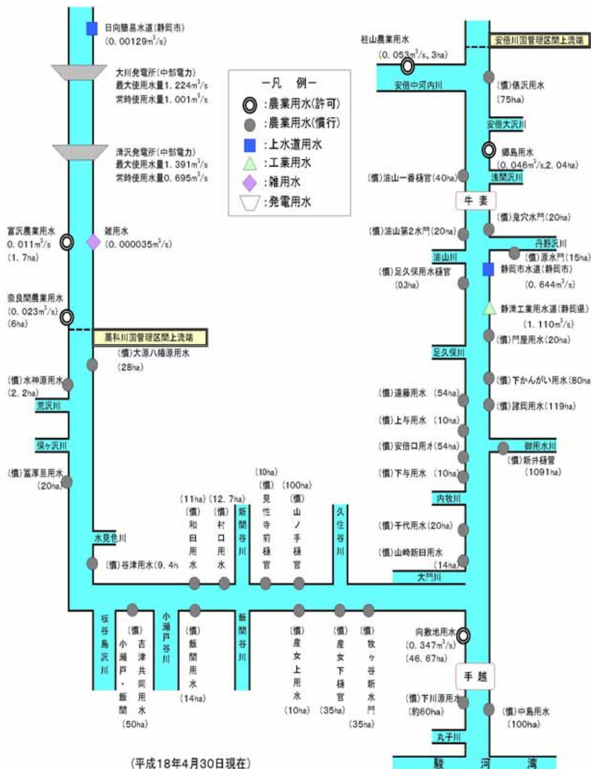
図-1.1.24 安倍川水利模式図
