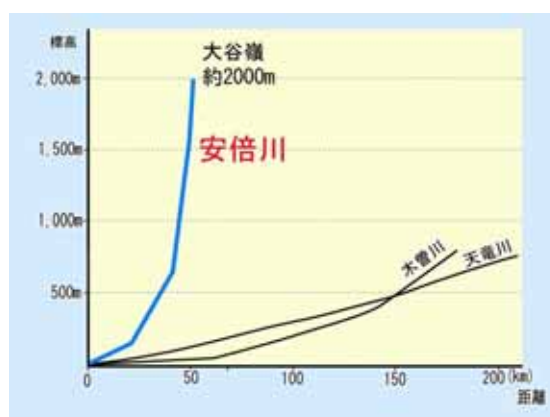
図-1.1.4 安倍川と中部地方の主要河川の縦断面図
