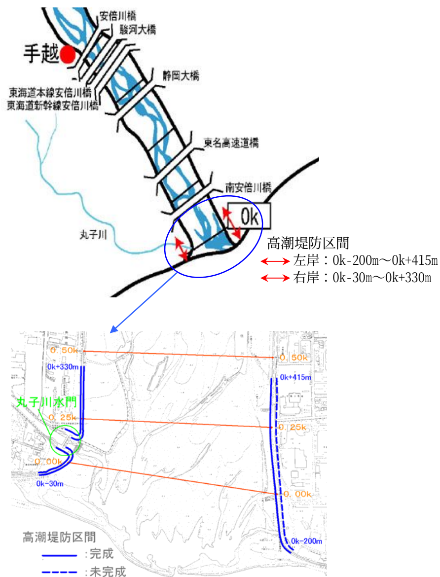
図-2.1.4 高潮堤防区間図
