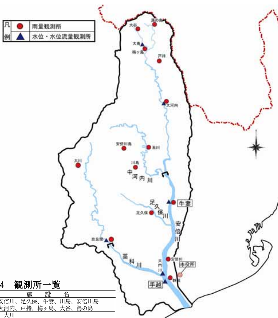
図-4.3.8 安倍川水系雨量・水位・流量観測所設置位置図
