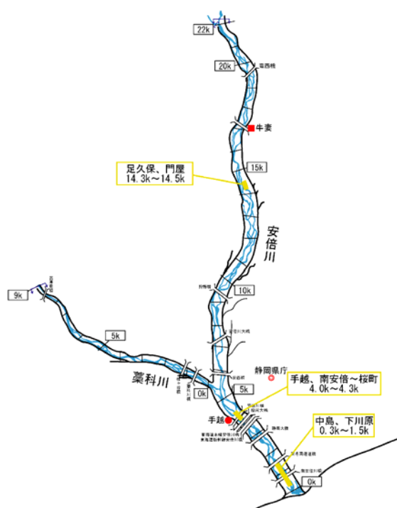
図-4.2.2 河道掘削に係る施行の場所
