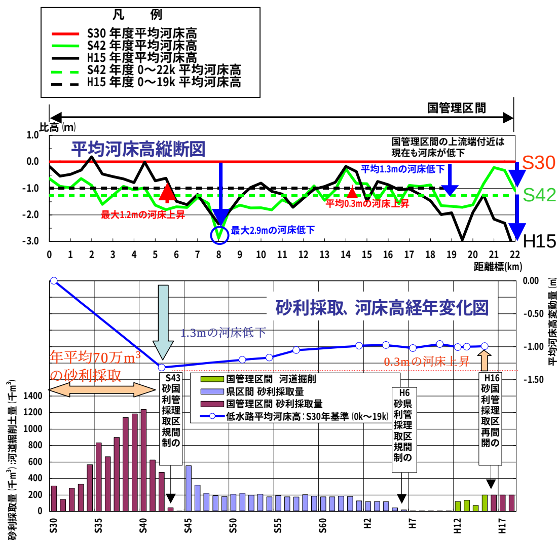
図-1.1.18 安倍川における砂利採取量及び低水路平均河床高 (国管理区間 0.0k~22.0k)
