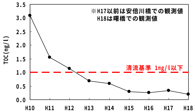
図-2.1.31 安倍川の TOC 経年変化図
