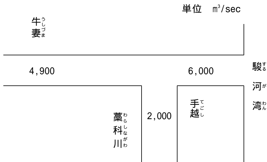
安倍川計画高水流量図
