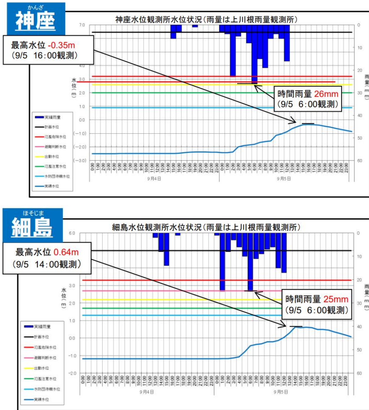
図-5 令和7年9月出水における雨量・水位
