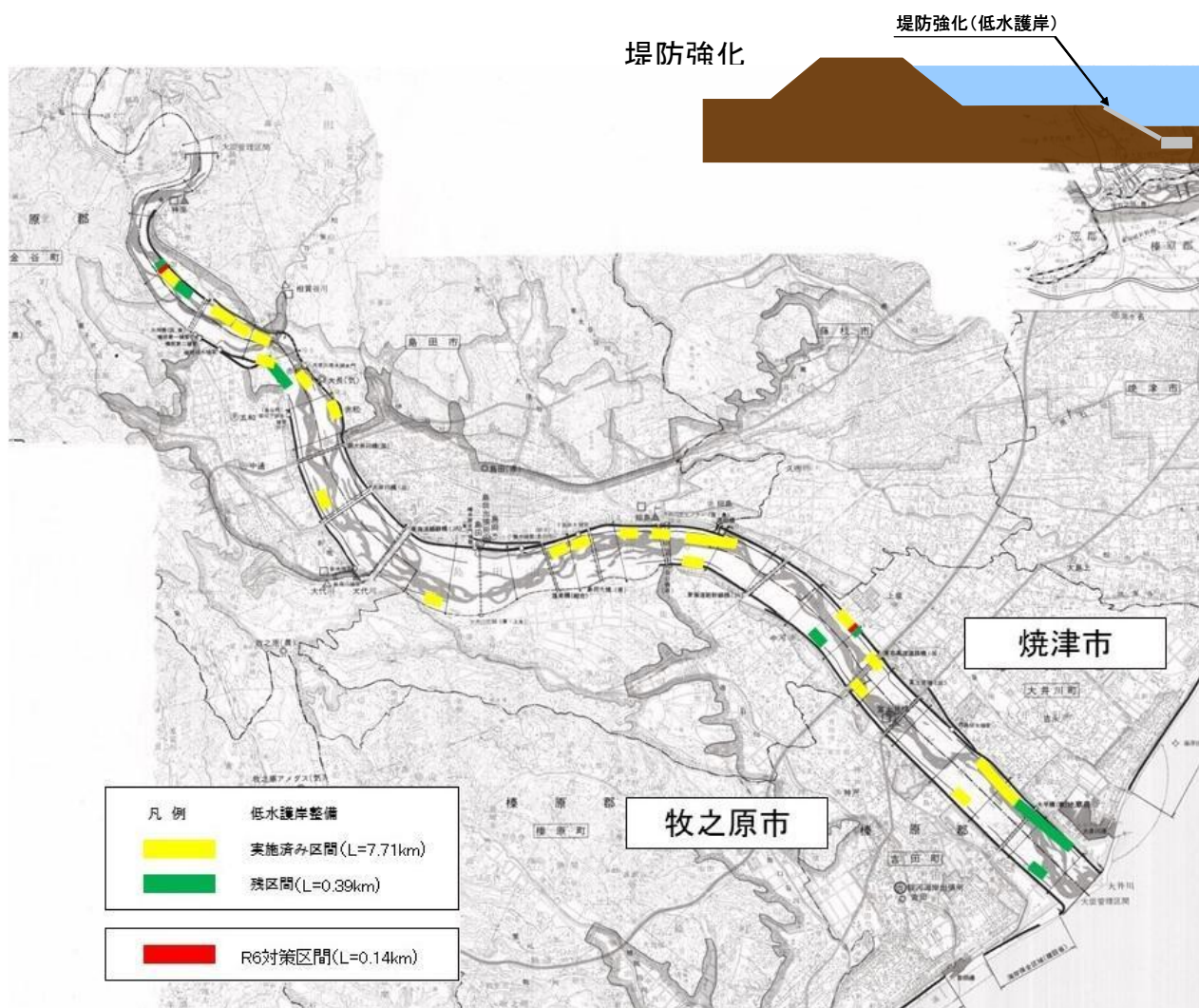
図-23 堤防強化対策実施状況
