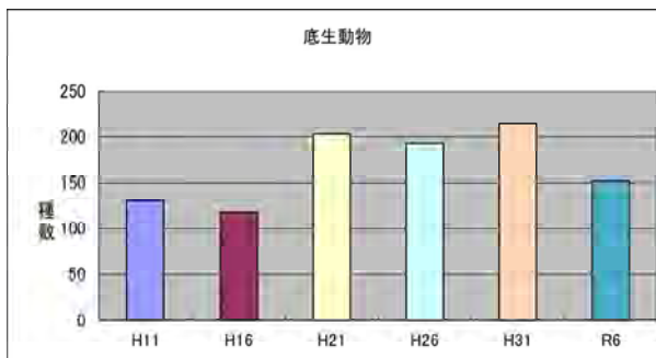
図-27 底生動物の変化
