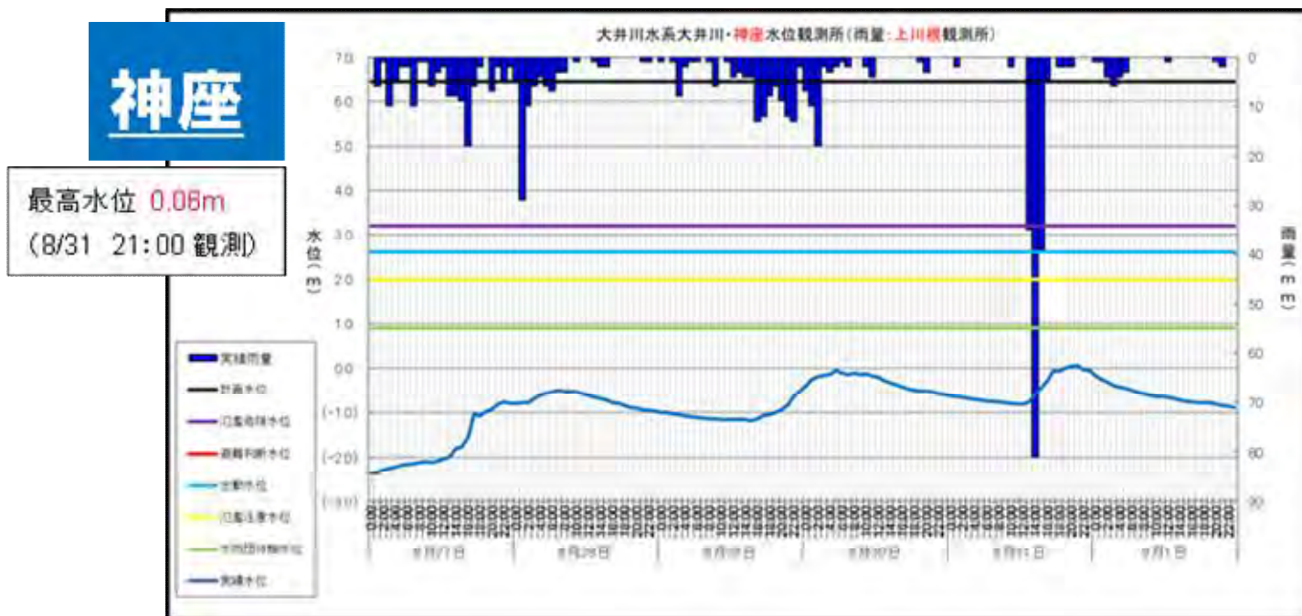
図-5 令和6年8月出水における雨量・水位
