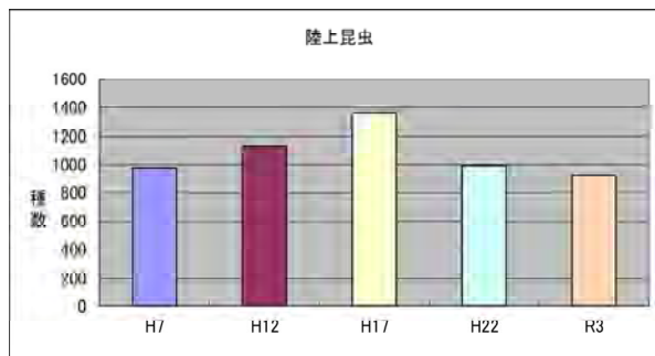
図-31 陸上昆虫の変化
