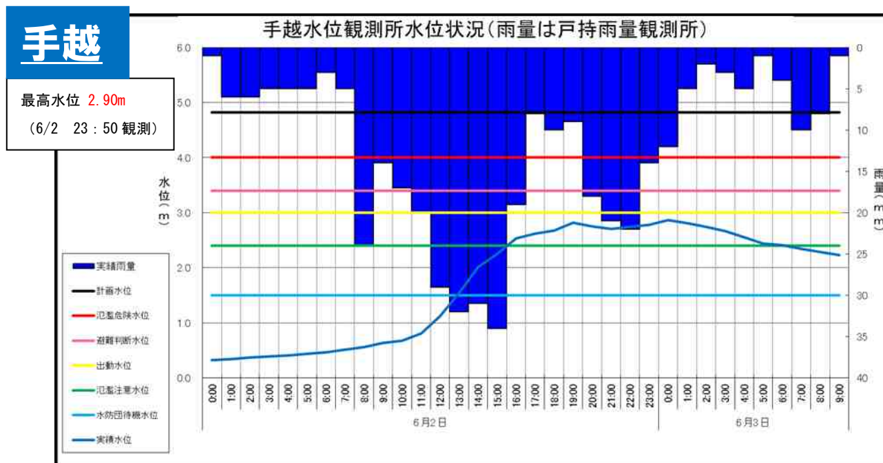
図-5 令和5年6月出水による雨量・水位
