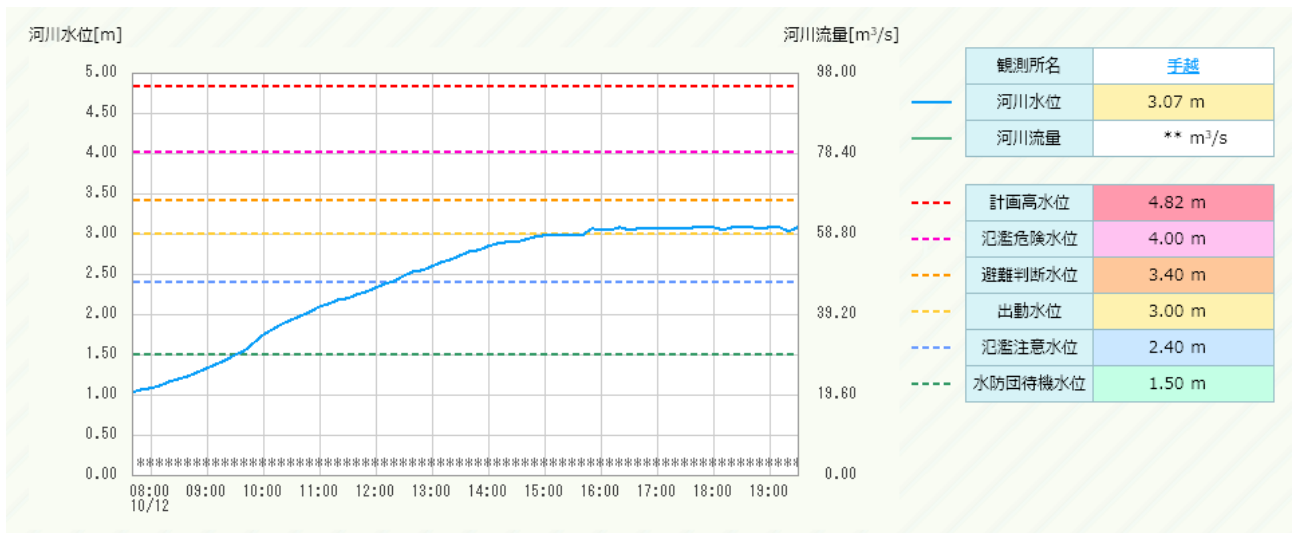
手越観測所水位グラフ
