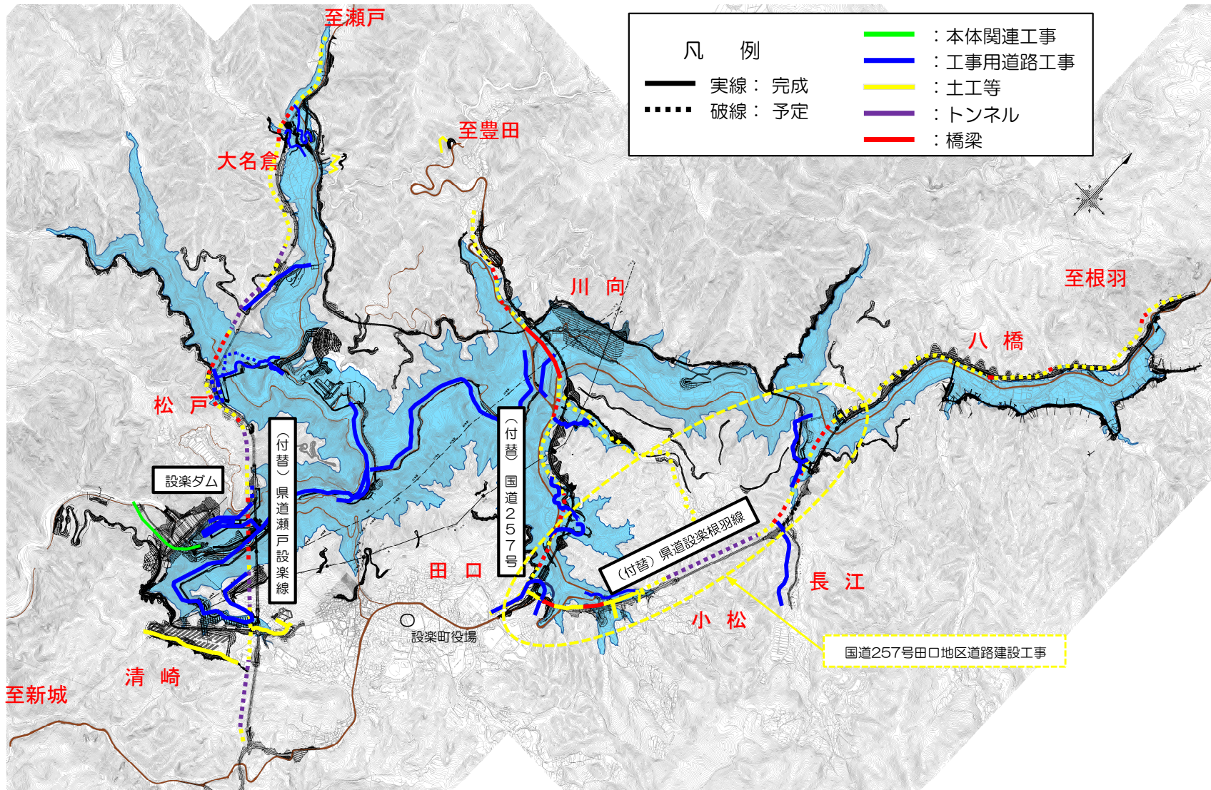
滝瀬橋～町道大野線～土工7工区
