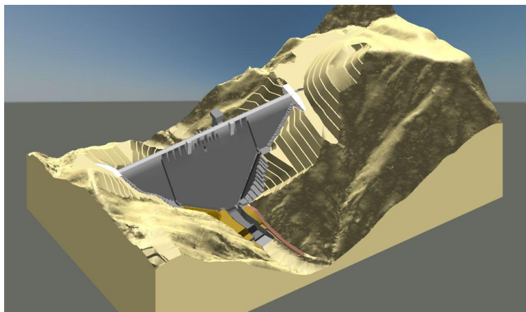
③設楽ダム本体3次元モデル
