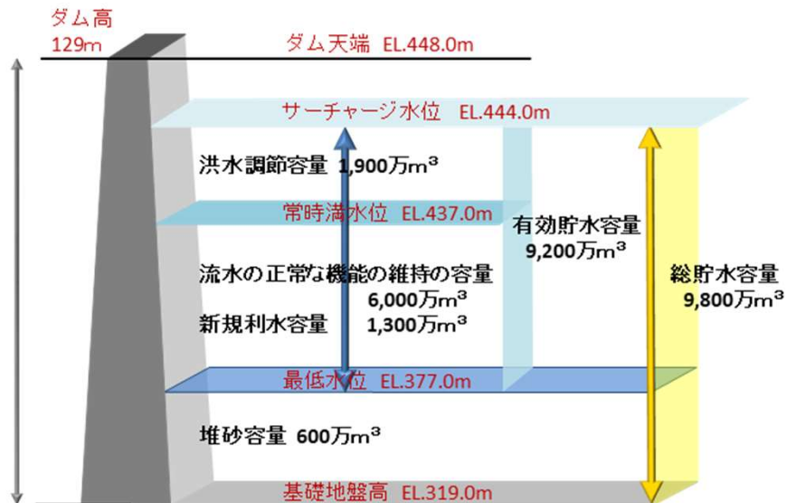
容量配分図
