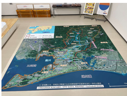
水の流れが分かる 豊川流域圏の衛星写真
