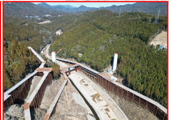
④5号橋PC上部工
