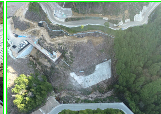
⑤清崎地区貯水池斜面对策
