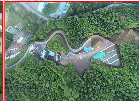
③2号橋右岸下部工
