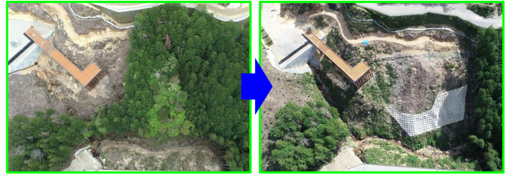
④令和4年度 設楽ダム清崎地区貯水池斜面对策工事 (令和6年9月完成)
