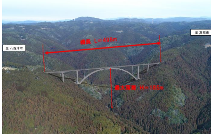
付替国道418号8号橋(仮称)工事現場視察の様子
