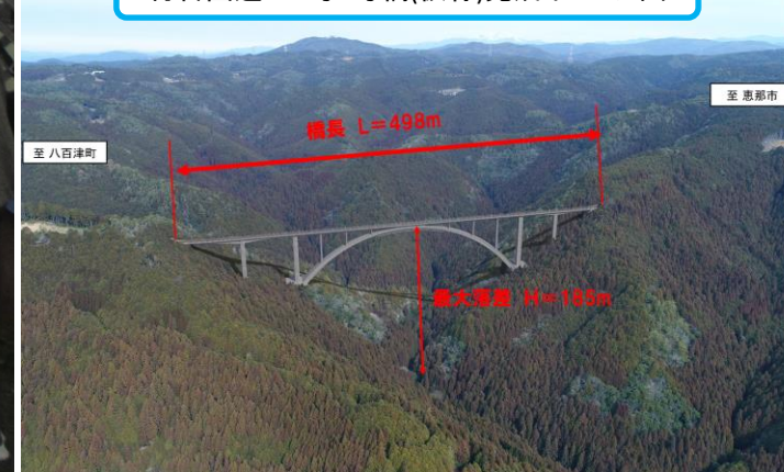
付替国道418号7号橋(仮称)完成イメージ図
