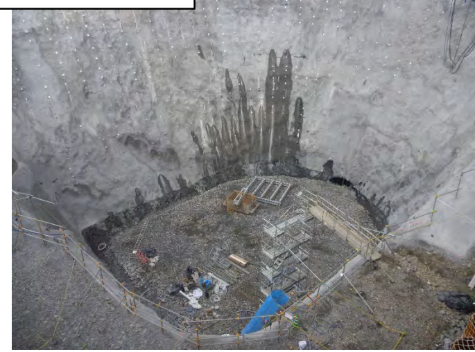
転流工の工事状況を見学
