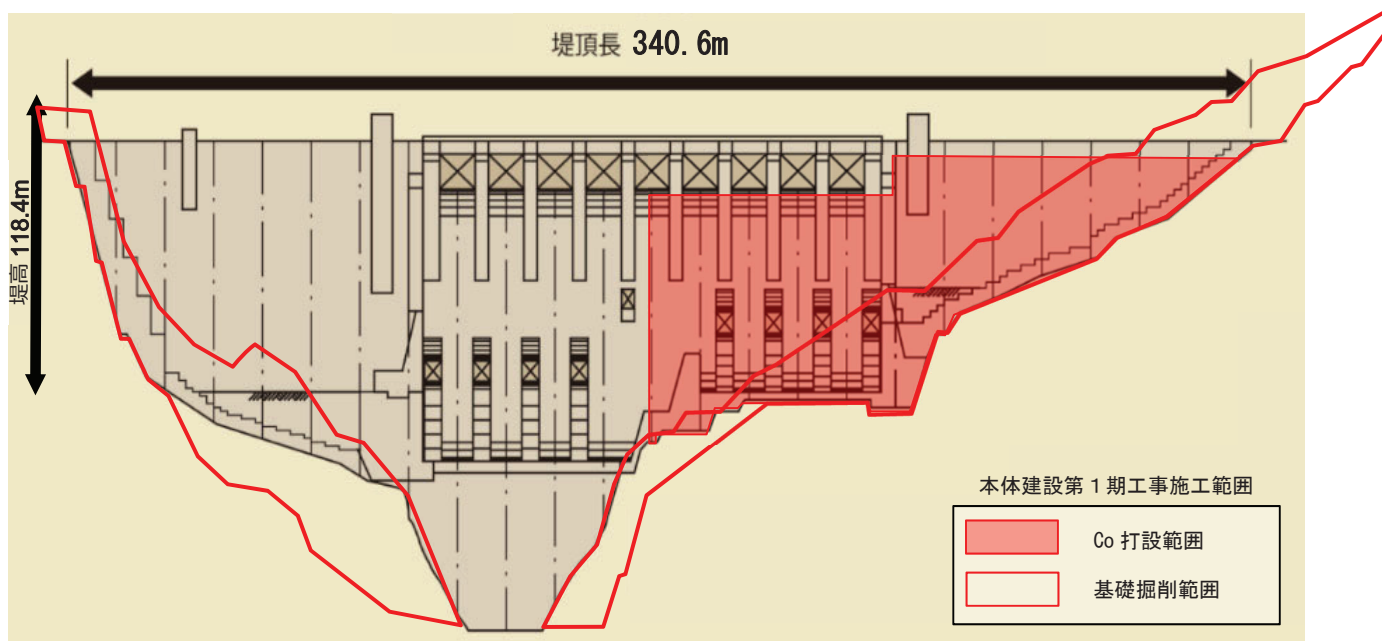
ダム下流図面
