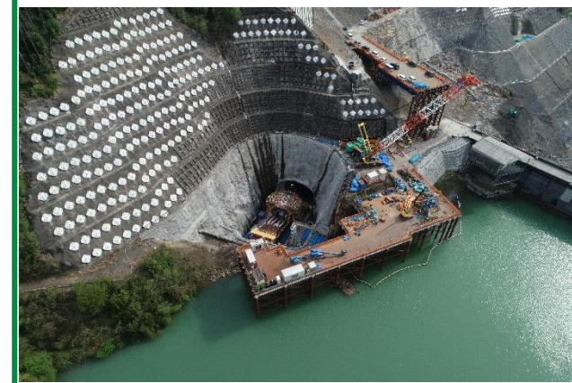
④ 転流工呑口部
