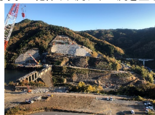
写真A 堤体(下流より上流を望む)
