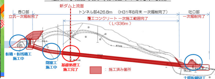
転流工事進捗状況（令和2年10月末時点）
