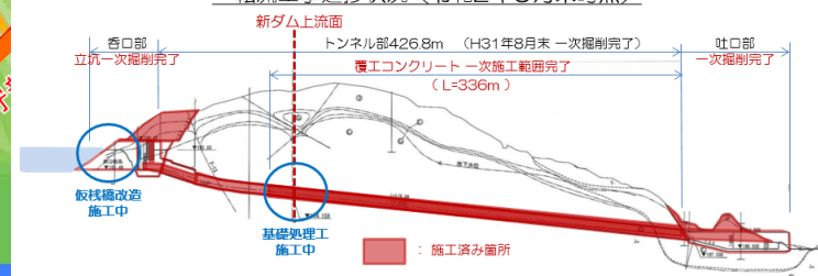
転流工事進捗状況(令和2年8月末時点)
