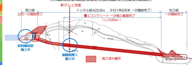
転流工事進捗状況（令和2年7月末時点）
