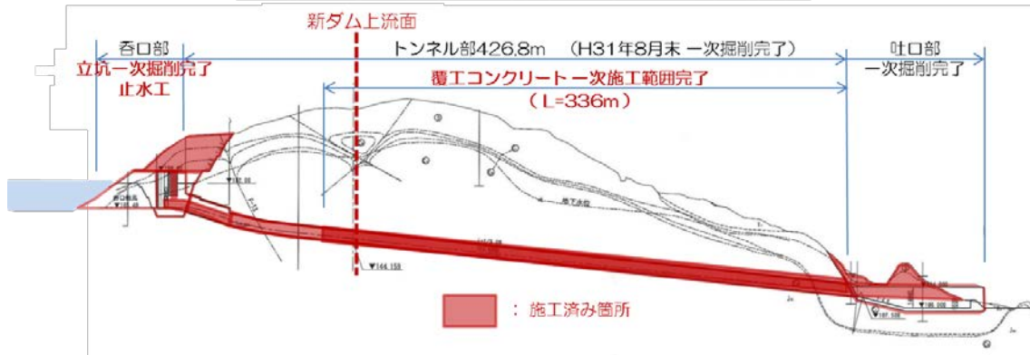
転流工事進捗状況 (令和元年11月末時点)
