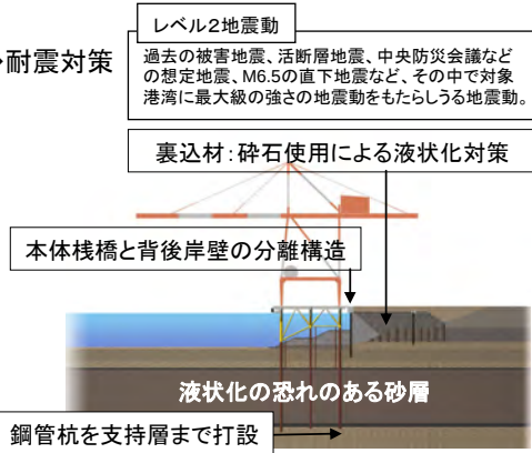
ジャケット式栈橋による大水深16m岸壁(耐震強化)イメージ (H17年12月、H20年12月供用)
