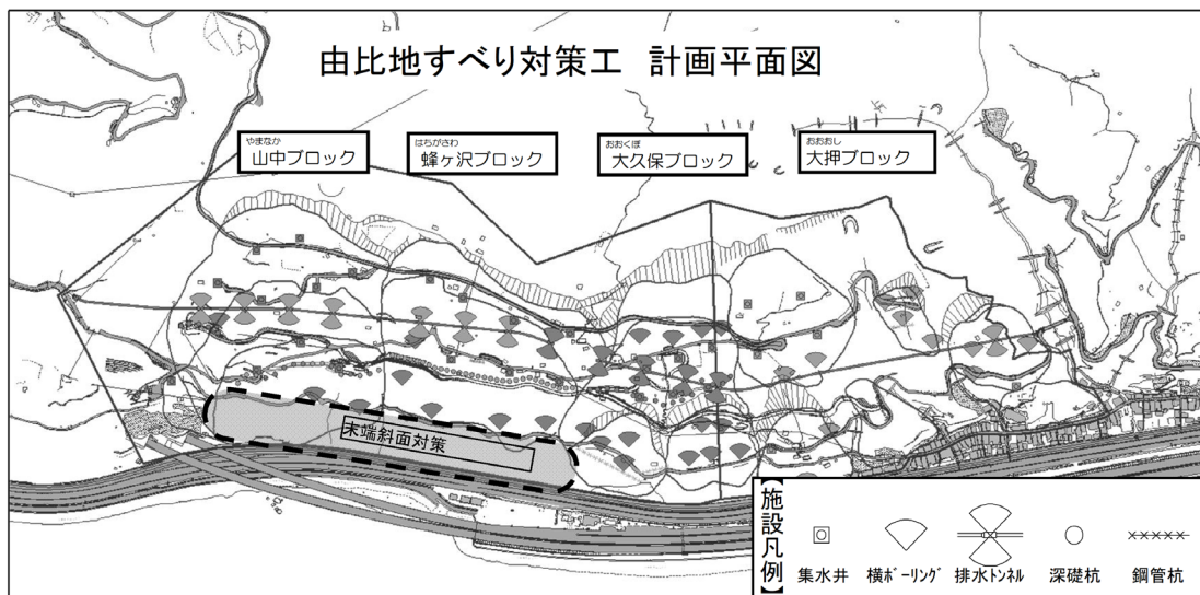
◇由比地区地すべり対策事業について
