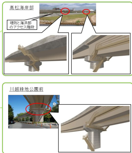
◇臨港道路の一時避難施設としての活用イメージ (四日市港霞4号幹線)
