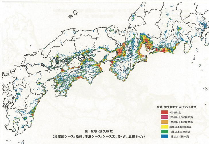
◇図 全壊・焼失棟数 (地震動ケース：陸側、津波ケース：ケース①、冬・夕、風速 8m/s)
