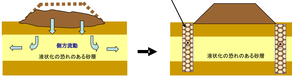
◇河川堤防の液状化対策
