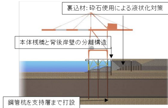
◇耐震強化岸壁の整備事例 (名古屋港)
