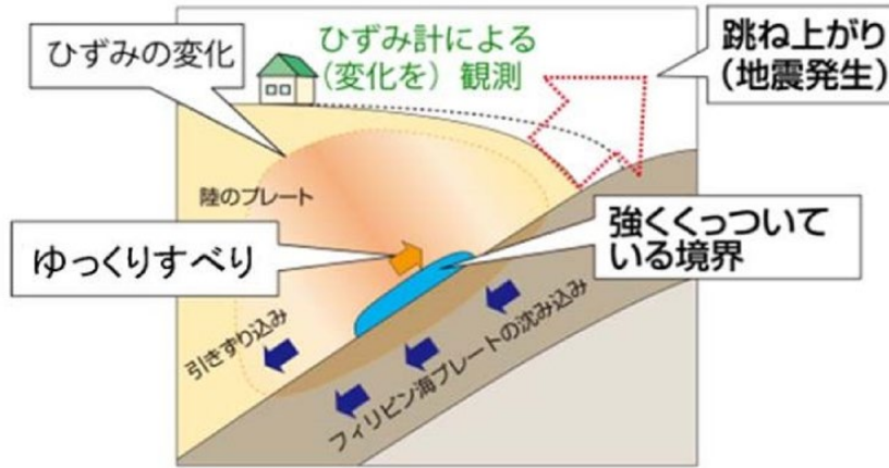
◇ゆっくりすべりのイメージ
