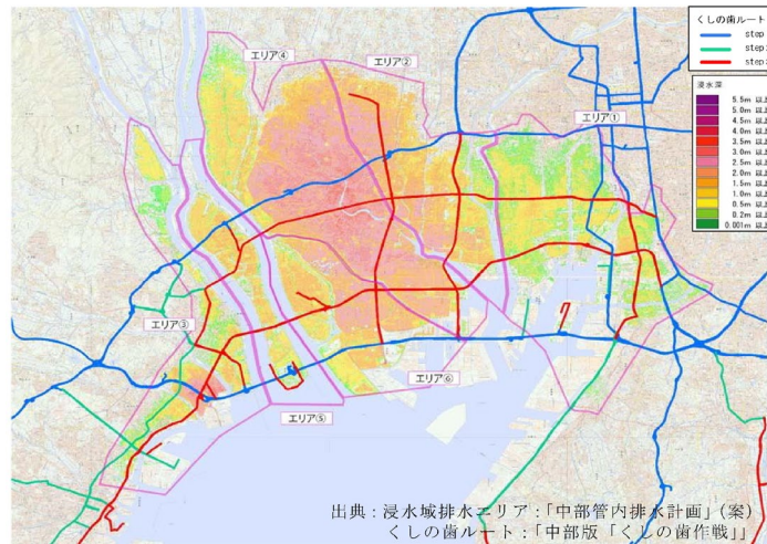
◇排水エリア図
