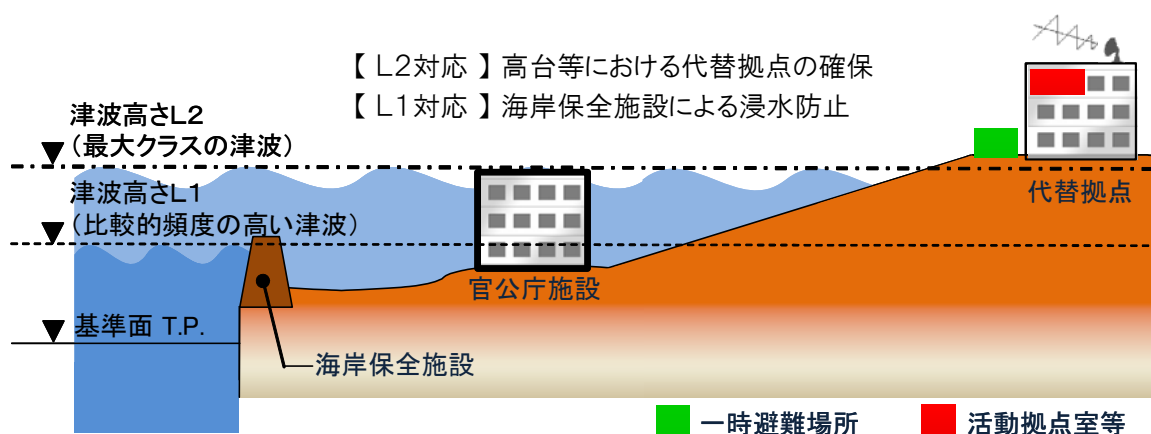
津波被害を想定した施設機能の確保【例】
