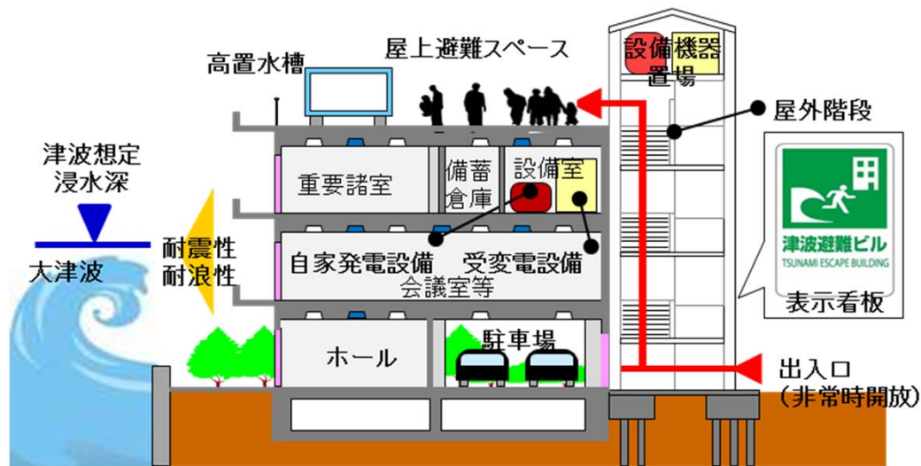
津波被害を想定した施設整備上の対策【例】
