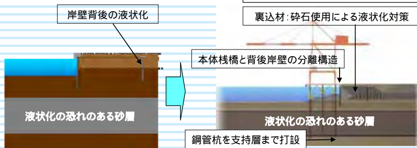
名古屋港における耐震強化護岸
